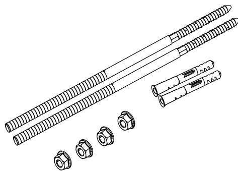
Шпильки крепления рамы M10 L — 250 мм
